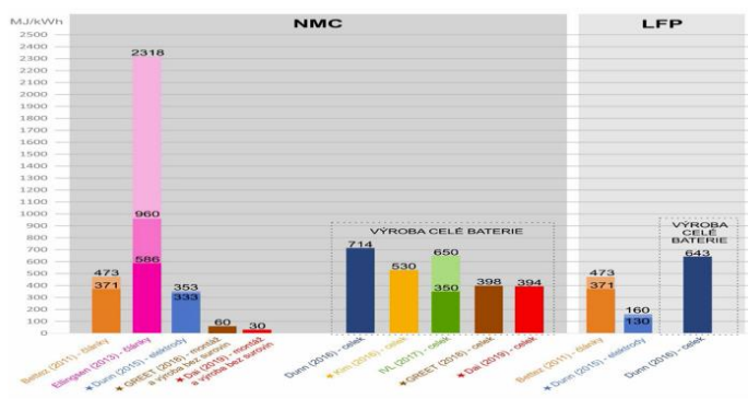
Obr. 8: Poměrná spotřeba elektrické energie na výrobu Li-ion NMC baterie [54]. Světlejší odstíny barev ukazují rozptyl hodnot
