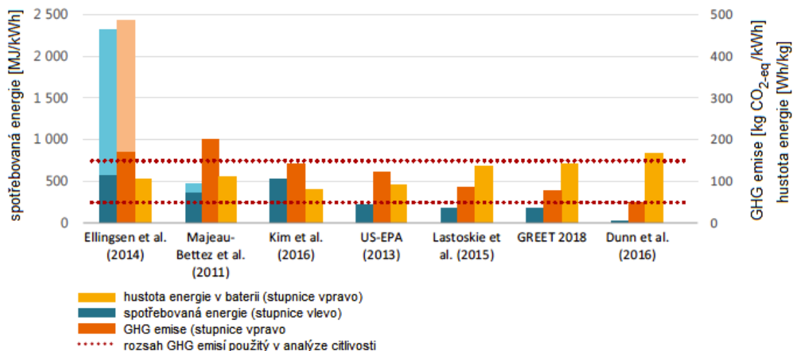
Obr. 7 Spotřebovaná energie a emise skleníkových plynů při výrobě NMC baterií a hustota energie v bateriích podle jednotlivých studií[4]. Světlejší odstíny barev ukazují rozptyl hodnot
