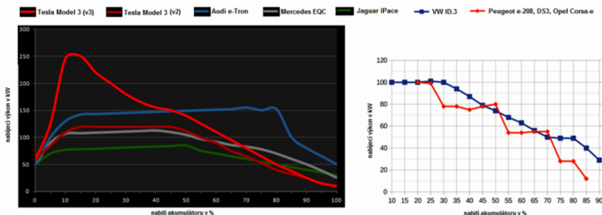
Obr. 10 Nabíjecí křivky [39], [40]
